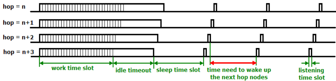
唤醒最坏情况示意图
