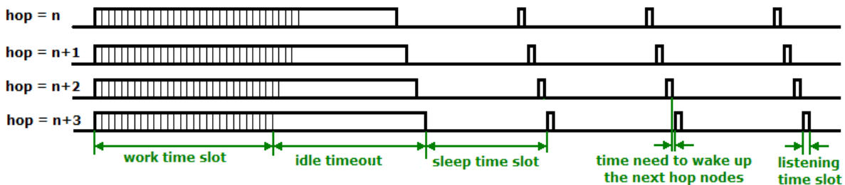
唤醒最理想情况示意图
