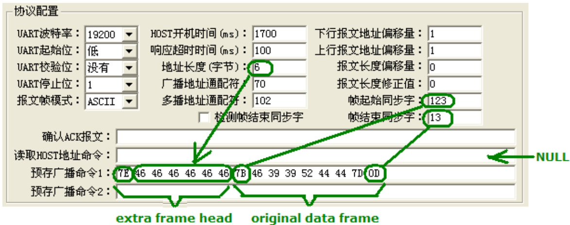
采用 MAC 地址配置示意图
