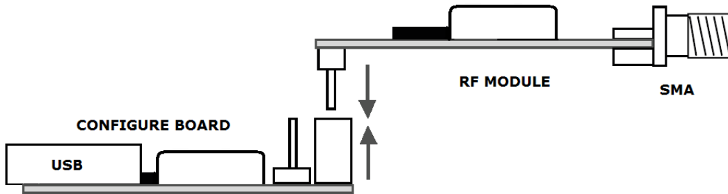
模块和配置板的连接示意图
